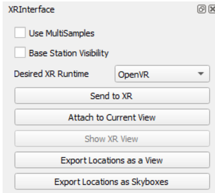
Fig. 1.54: XRInterface panel.
